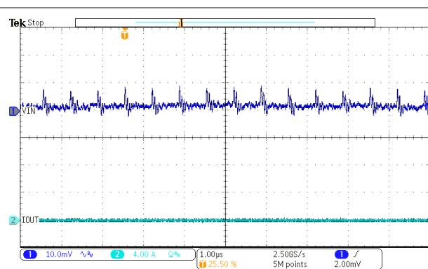
7-17. Input Ripple – No Load
