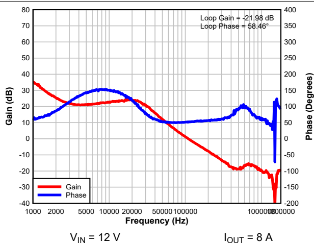
図 7-7. Bode Plot
