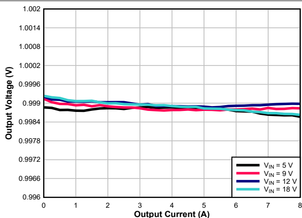
図 7-5. Load Regulation
