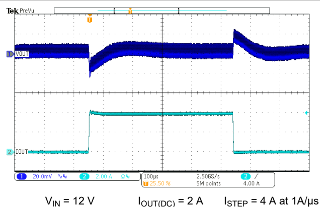
図 7-8. Load Transient
