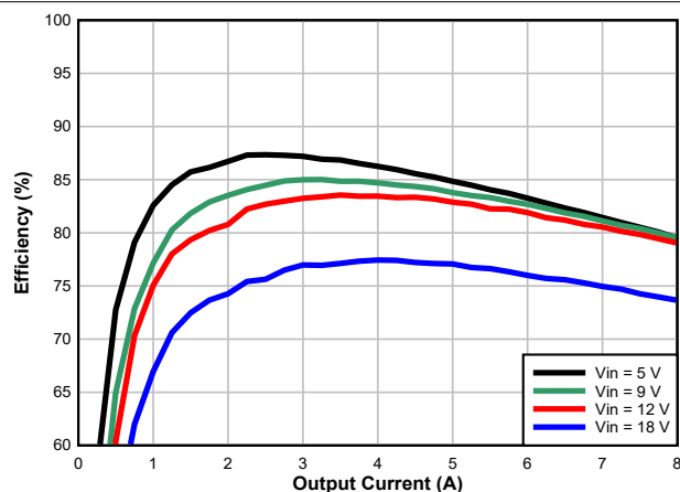
図 7-4. Efficiency
