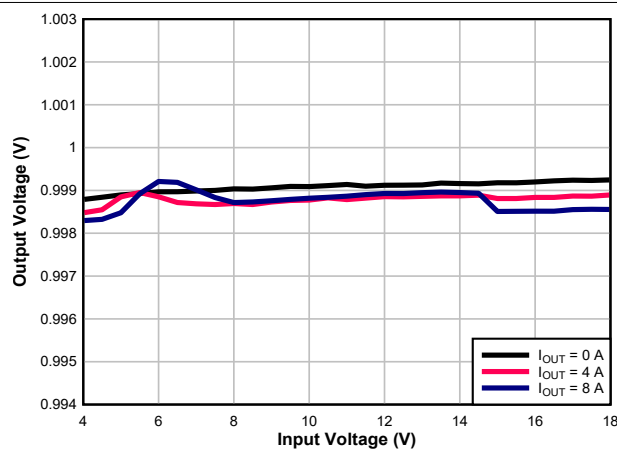
図 7-6. Line Regulation
