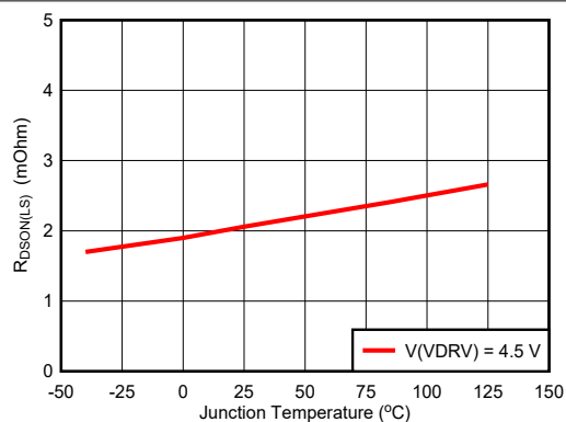
图 6-2. Low-Side FET R_{DS(ON)}
