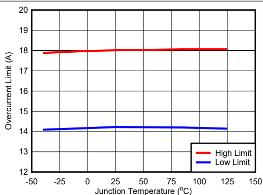
图 6-3. Overcurrent Limit
