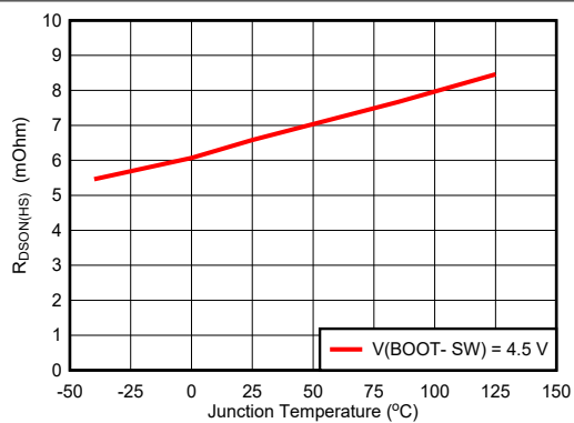
图 6-1. High-Side FET R_{DS(ON)}
