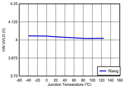
图 6-7. V_{IN} UVLO
