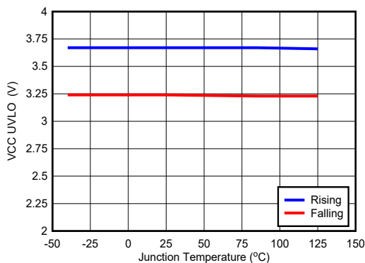
图 6-8. V_{CC} UVLO
