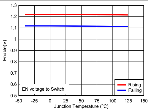
图 6-5. Enable Voltage
