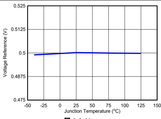
6-6. VREF
