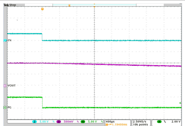
図 8-10. EN Shutdown
