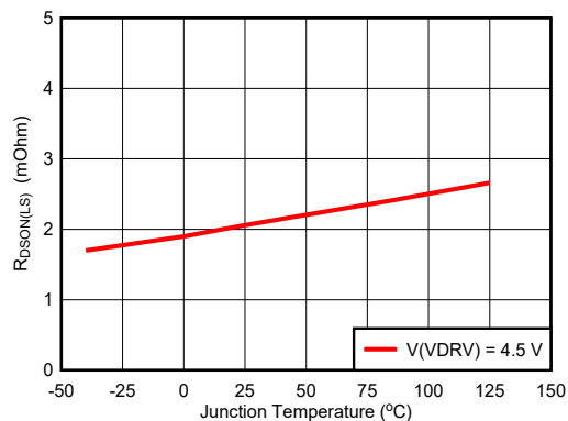
6-2. Low-Side FET RdsON
