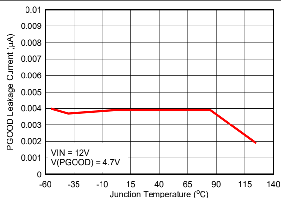
图 6-10. PG Leakage Current
