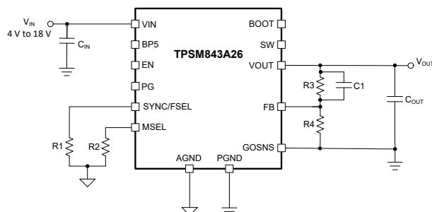
TPSM843A26E のアプリケーション概略図
