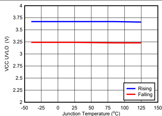
图 6-8. V_{CC} UVLO
