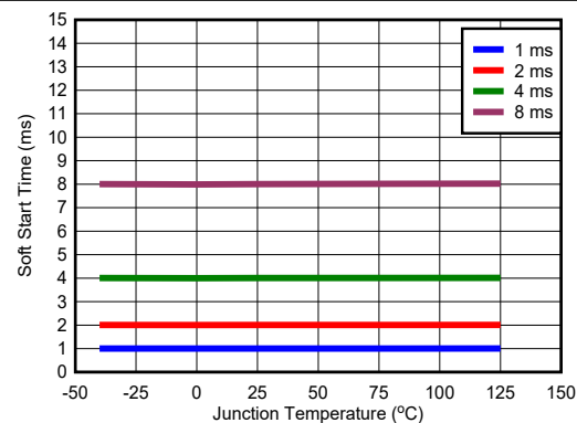
图 6-12. Soft Start
