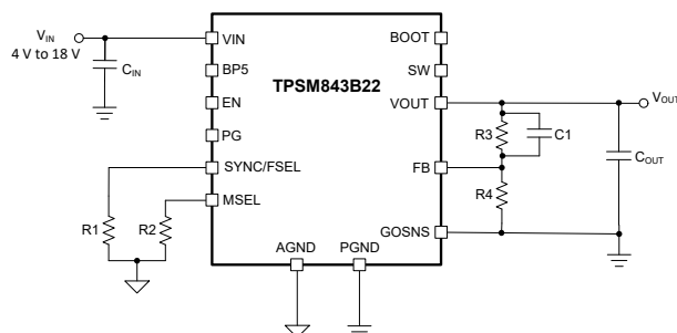
TPSM843B22 のアプリケーション概略図
