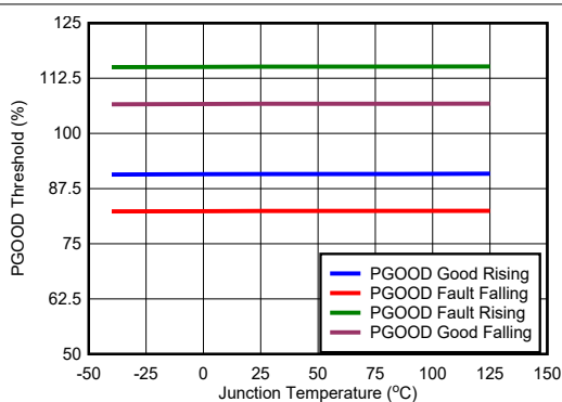
图 6-9. PG Threshold
