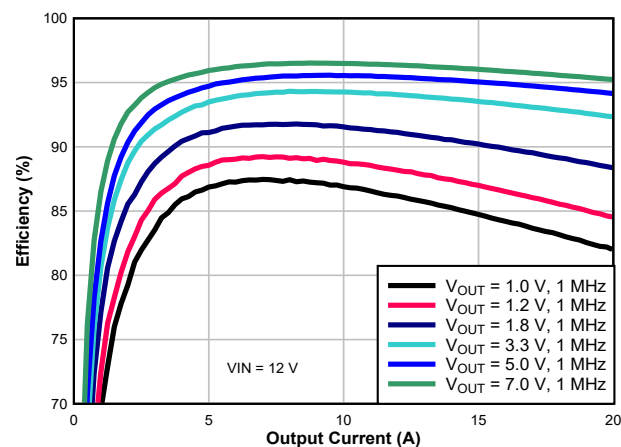
代表的なアプリケーションの効率
