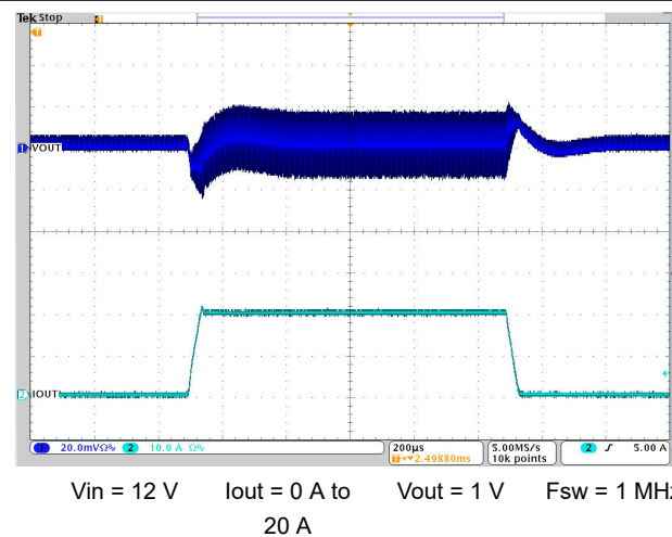
图 8-8. Load Transient
