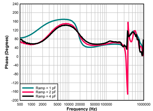
図 7-7. Loop Phase vs Ramp Settings
