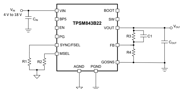
TPSM843B22E のアプリケーション概略図
