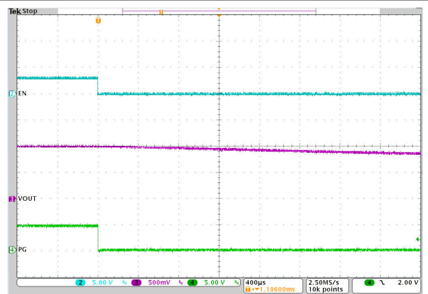
図 8-10. EN Shutdown
