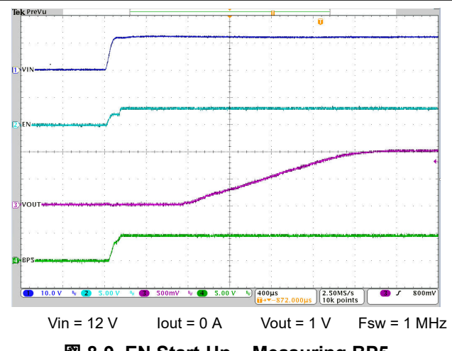
图 8-9. EN Start-Up – Measuring BP5
