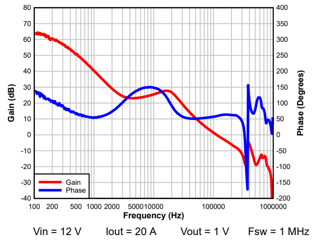
图 8-7. Bode Plot
