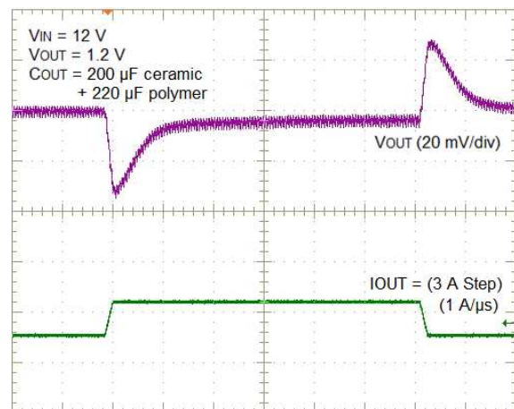
過渡応答
