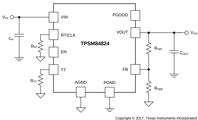
概略回路図
