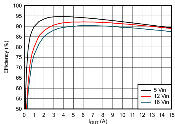
图 8-4. Efficiency
