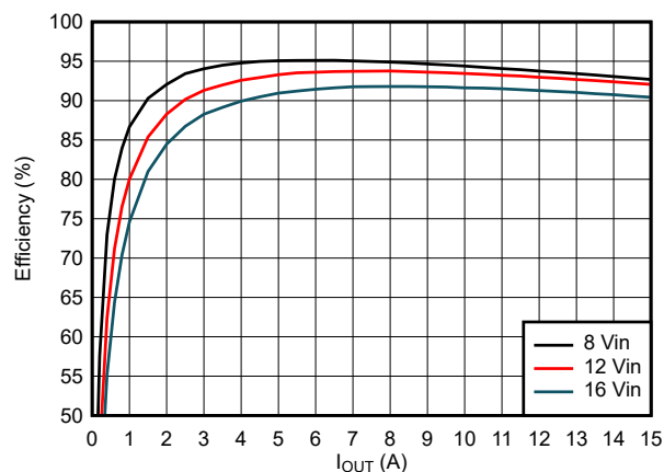
图 8-6. Efficiency
