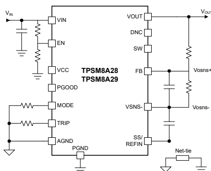
概略回路図
