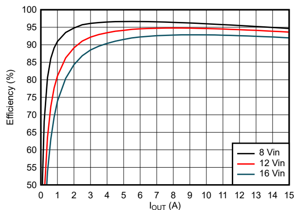
图 8-7. Efficiency
