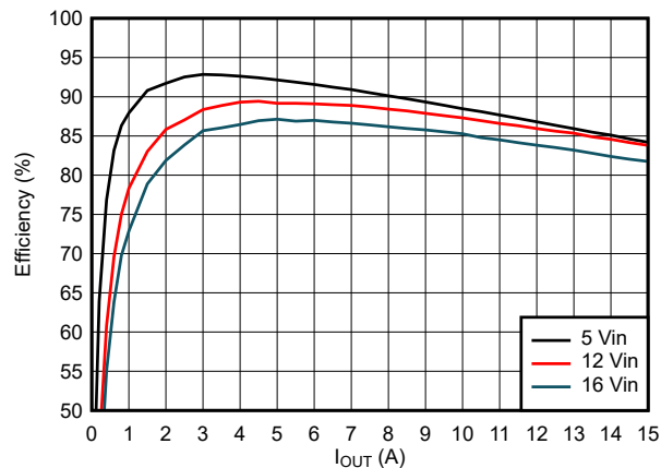
图 8-4. Efficiency
