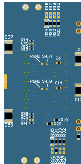
図 8-20. 最下層部品 (上面図)
