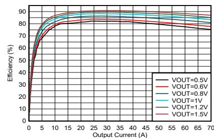
効率、12Vin、内部バイアス、F sw = 550kHz
