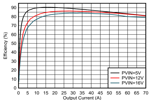
図 8-10. 効率と出力電流との関係
