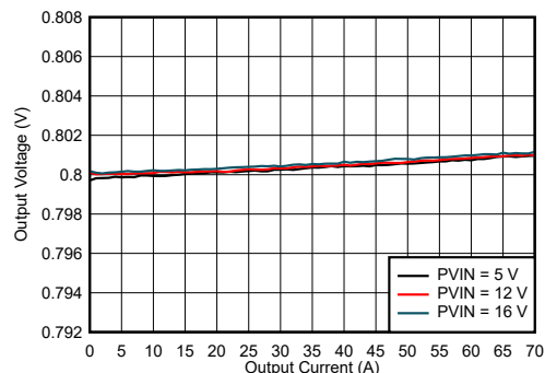
図 8-11. ロードレギュレーション
