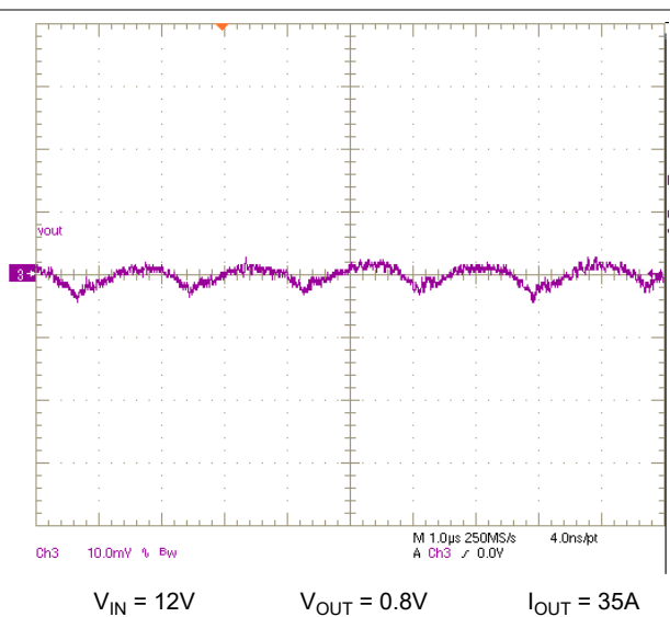
図 8-8. V_{OUT} 定常状態リップル
