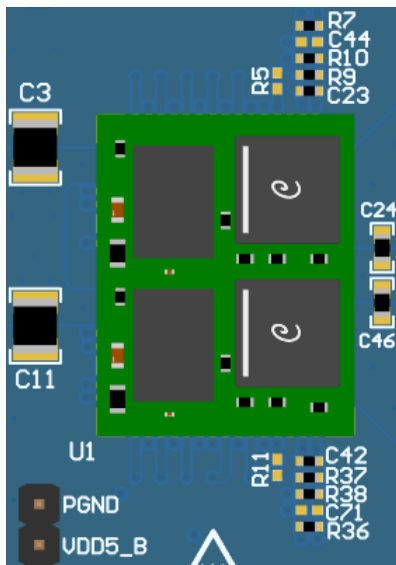
図 8-19. 最上層部品 (上面図)
