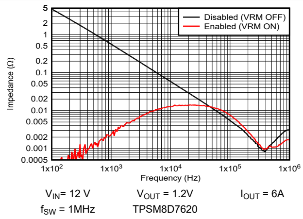
図 8-11. VOUT2 の出カインピーダンス
