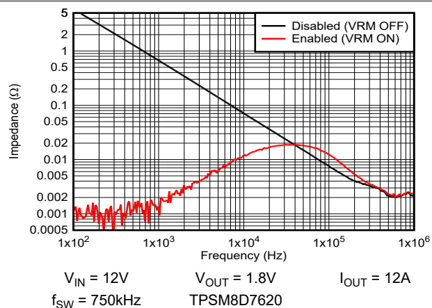
図 8-24. VOUT1 の出力インピーダンス
