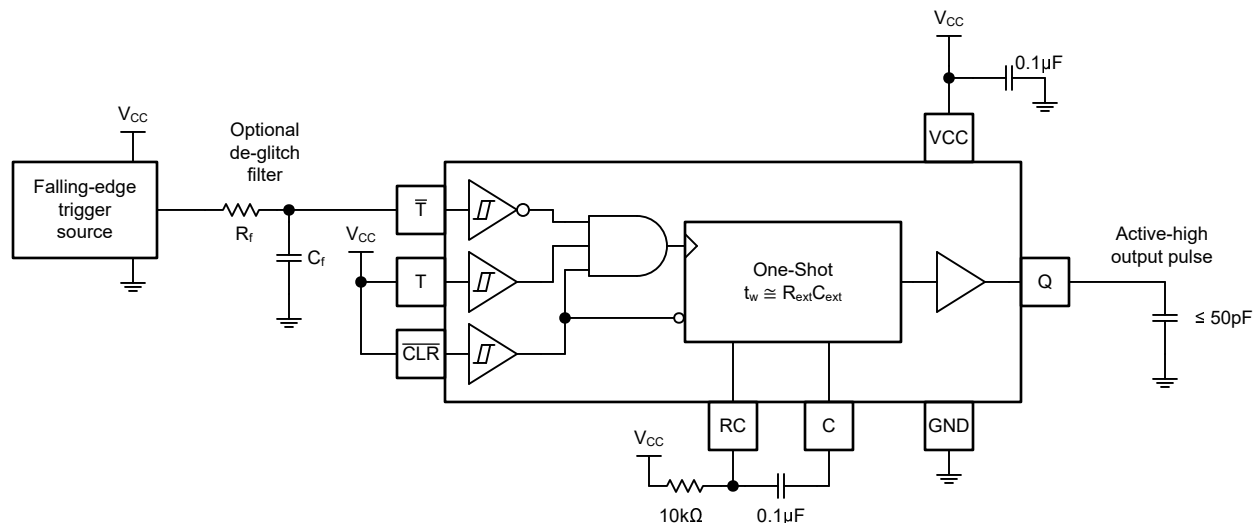
図 8-1. TPUL1G113-Q1 を使用したパルス生成
