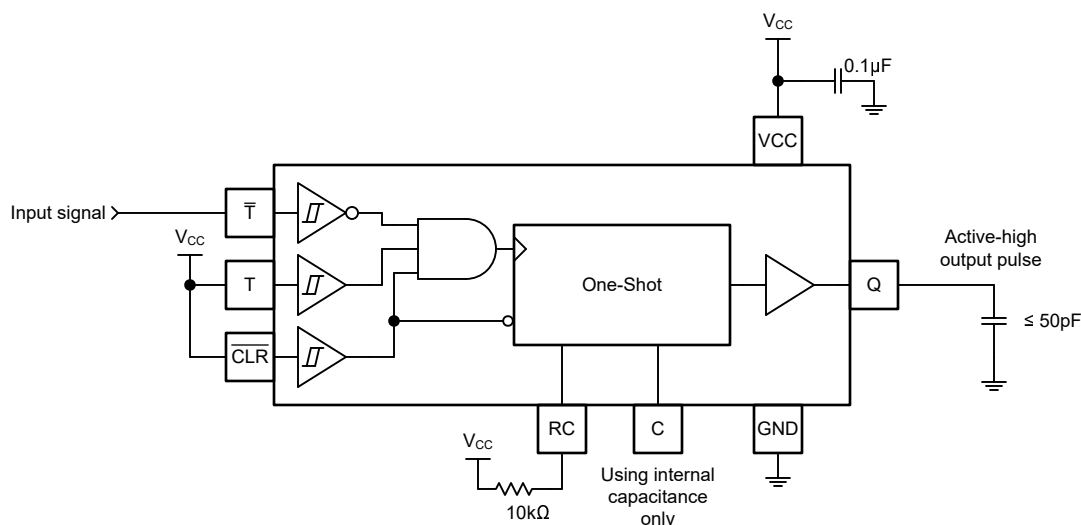
図 8-4. TPUL1G113-Q1 を使用した立ち下がりエッジ検出
