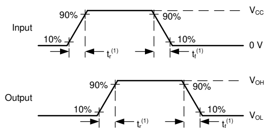
図 6-3. 電圧波形、入力および出力の遷移時間
