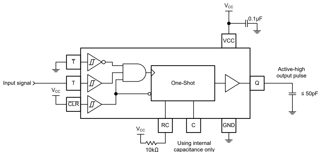
図 8-3. TPUL1G113-Q1 を使用した立ち上がりエッジ検出
