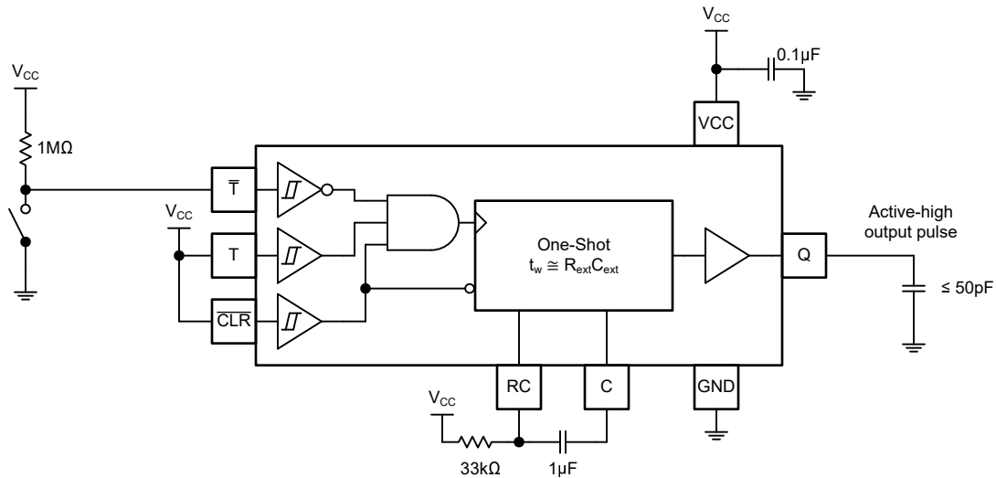
図 8-5. TPUL1G113-Q1 を使用した、スイッチのデバウンス
