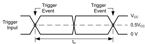
図 6-4. 電圧波形、リトリガ時間
