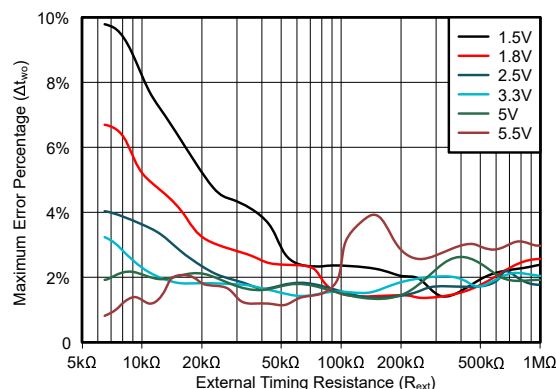
図 5-23. C_{\text{ext}} = 100\text{pF} の最大出力パルス幅誤差 (絶対値) とタイミング抵抗値との関係
