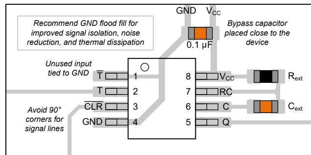
図 8-3. レイアウト例
