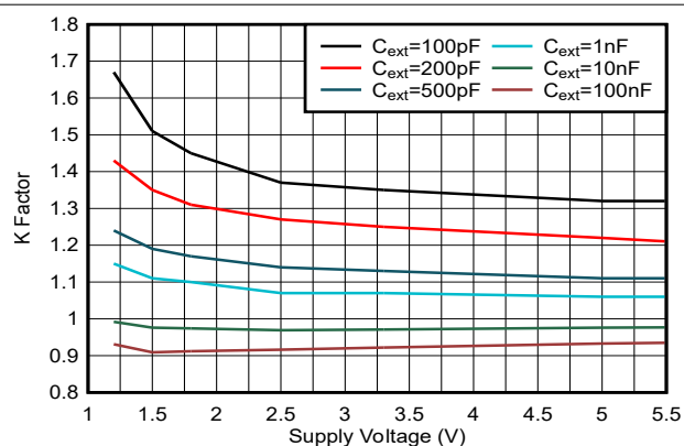
図 5-7. K 係数と電源電圧との関係、R ext = 10kΩ
