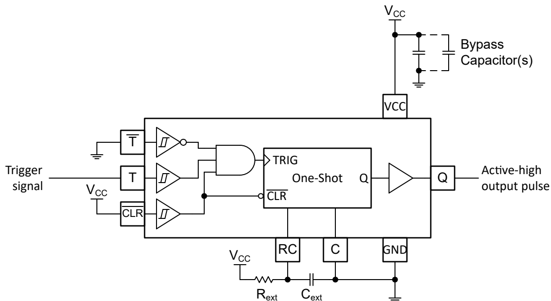
図 8-1. TPUL1G313-Q1 を使用したパルス生成
