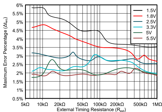
図 5-24. C_{\text{ext}} = 1\text{nF} の最大出力パルス幅誤差 (絶対値) とタイミング抵抗値との関係
