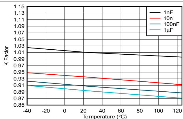
図 5-6. K 係数と温度との関係、R ext = 10kΩ
