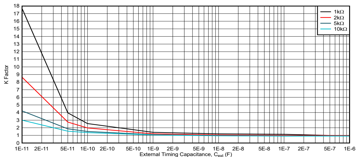
図 5-8. K 係数、V CC = 1.5V、R ext = 1kΩ ~ 10kΩ
