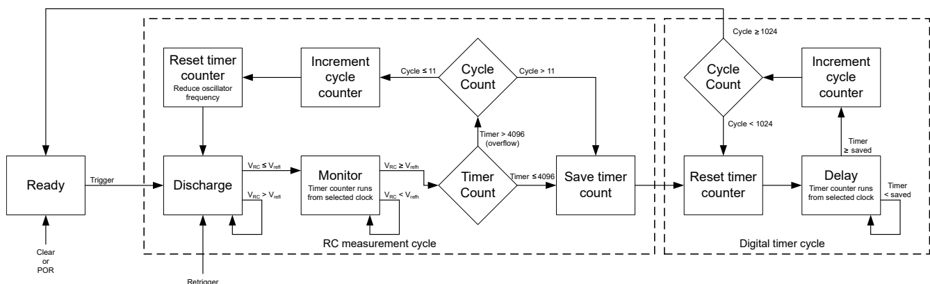
図 7-3. ステート マシンの図
