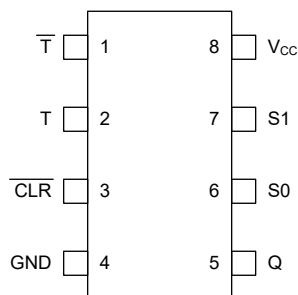
図 4-1. TPUL1G513-Q1 DRL パッケージ（上面図）
