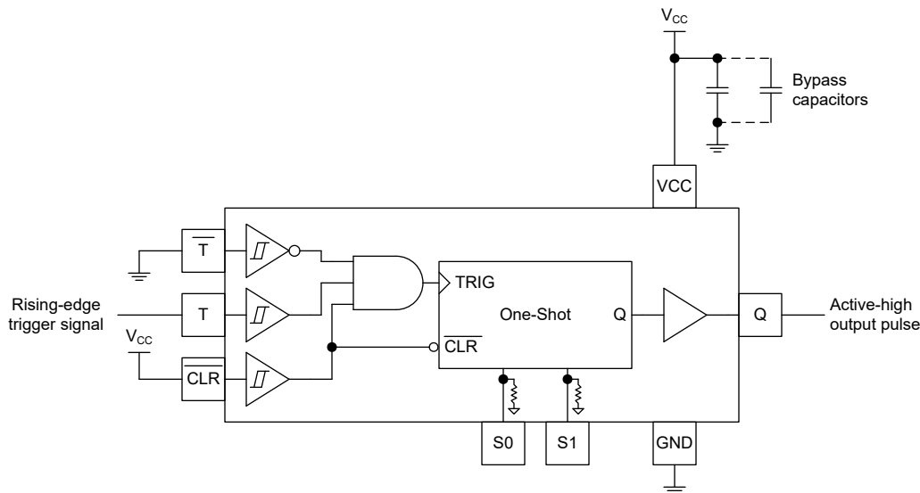
図 8-1. TPUL1G513-Q1 を使用したパルス ジェネレータの回路図
