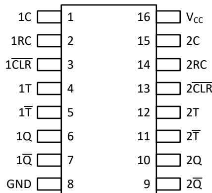
図 4-1. TPUL2G122 D および PW パッケージ 16 ピン SOIC および TSSOP 上面図 図 4-2. TPUL2G122A D および PW パッケージ 16 ピン SOIC および TSSOP 上面図
