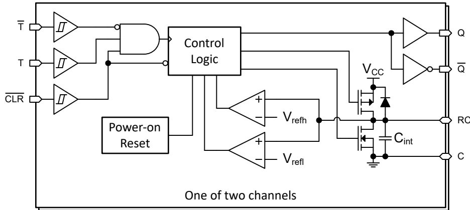
図 7-3. TPUL2G122
