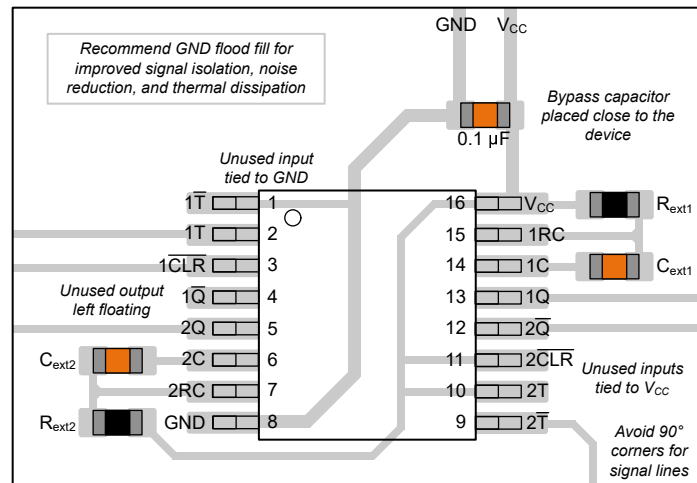
図 8-6. PW (TSSOP) パッケージの TPUL2G122x のプッシュプルレイアウト例
