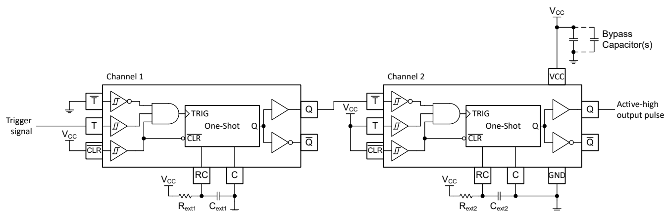
図 8-4. TPUL2G122x を使用した遅延パルス生成回路図
