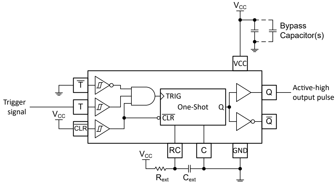
図 8-1. TPUL2G122x を使用したパルス ジェネレータの回路図
