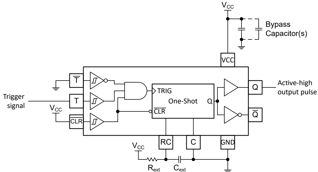
図 8-1. TPUL2G122x-Q1 を使用したパルス ジェネレータの回路図
