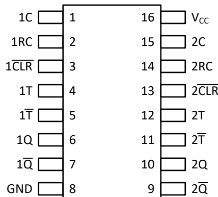
図 4-2. TPUL2G122A-Q1 D および PW パッケージ 16 ピン SOIC および TSSOP 上面図
