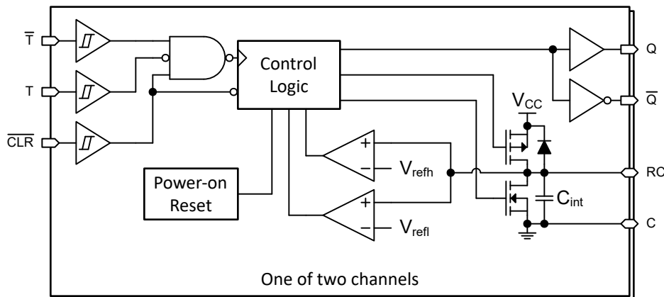
図 7-4. TPUL2G122A-Q1
