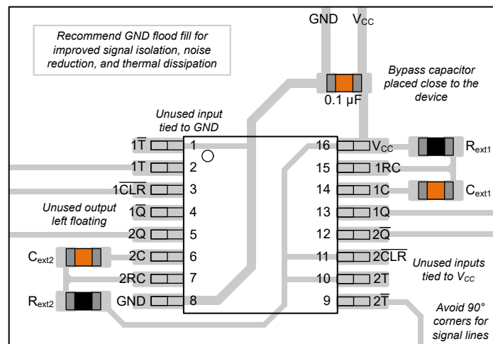
図 8-6. PW (TSSOP) パッケージの TPUL2G122x-Q1 のプッシュアップレイアウト例
