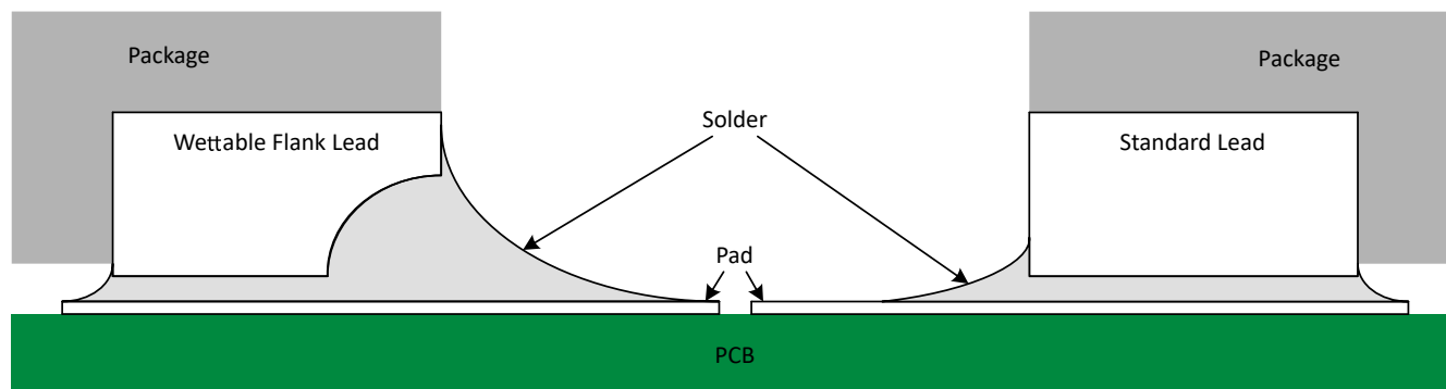
図 7-7. 半田付け後のウェッタブル フランク QFN パッケージと標準 QFN パッケージの概略断面図
