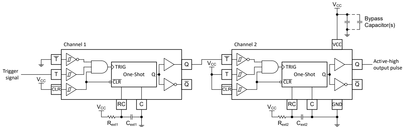
図 8-4. TPUL2G122x-Q1 を使用した遅延パルス生成回路図
