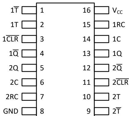
図 4-1. TPUL2G122-Q1 D および PW パッケージ 16 ピン SOIC および TSSOP 上面図
