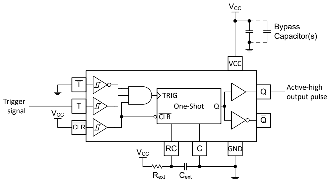
図 8-1. TPUL2G123 を使用したパルス ジェネレータの回路図
