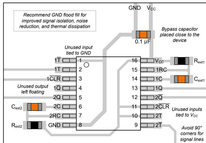
図 8-6. PW (TSSOP) パッケージの TPUL2G123 のプッシュプルレイアウト例
