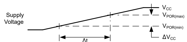
図 6-6. 電圧波形、電源ランプ
