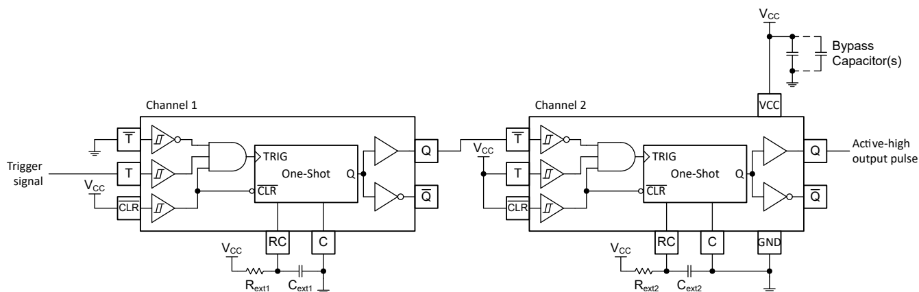
図 8-4. TPUL2G223 を使用した遅延パルス生成回路図
