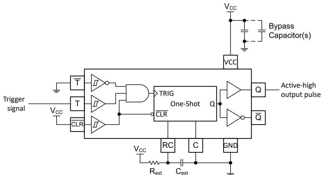
図 8-1. TPUL2G223 を使用したパルス ジェネレータの回路図
