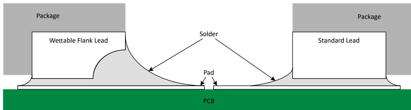
図 7-8. 半田付け後のウェッタブル フランク QFN パッケージと標準 QFN パッケージの概略断面図
