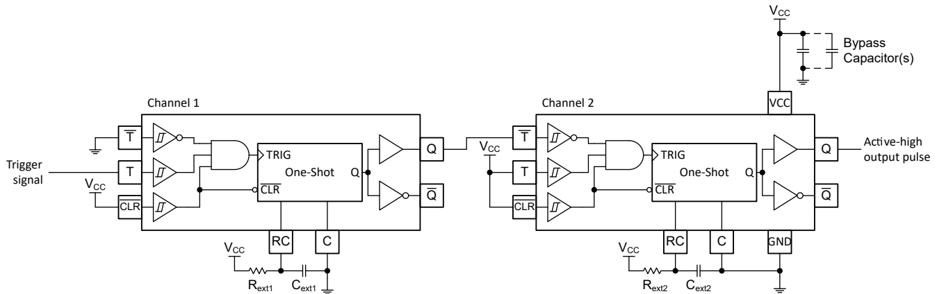
図 8-4. TPUL2T122x-Q1 を使用した遅延パルス生成回路図
