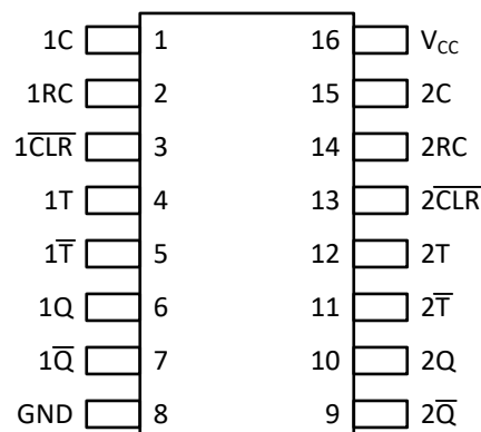
図 4-2. TPUL2T122A-Q1 D および PW パッケージ 16 ピン SOIC および TSSOP 上面図
