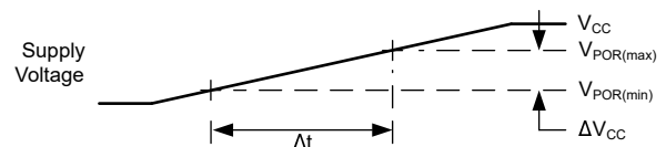
図 6-6. 電圧波形、電源ランブ
