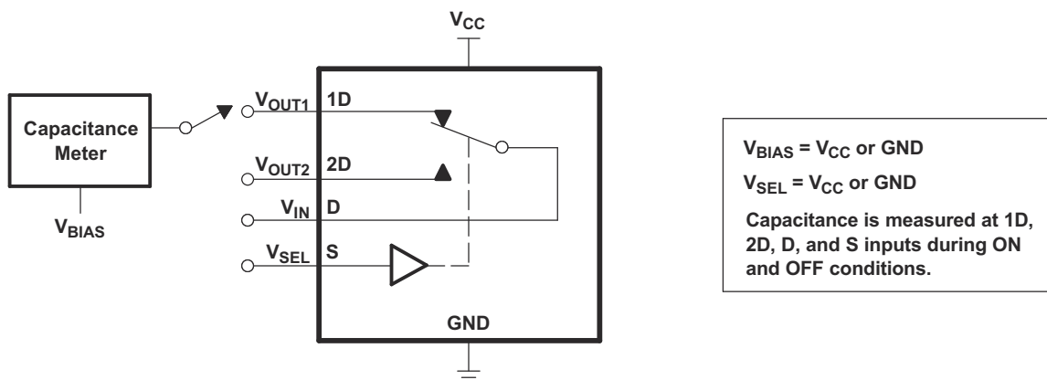
図 6-9. Capacitance
