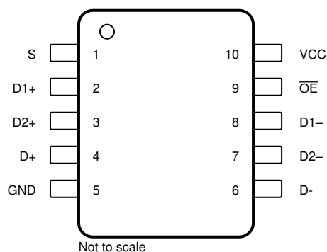
図 4-2. DGS Package 10-Pin VSSOP Top View
