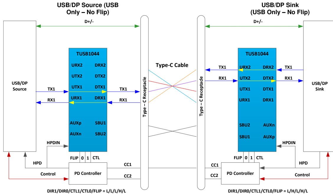
図 9-4. USB3.2 のみ – フリップ機能なし
