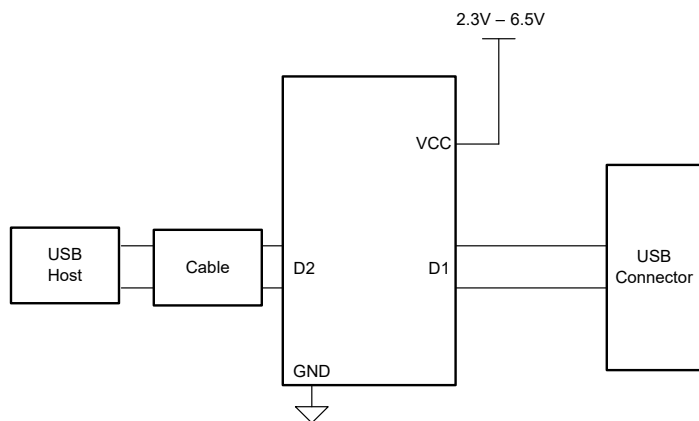
概略回路図
