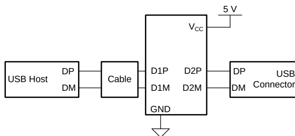
概略回路図
