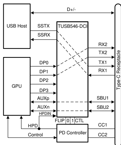
簡略回路図
