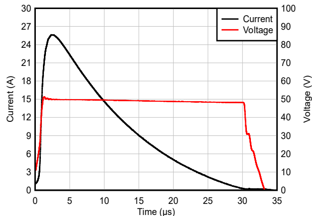
図 7-1. 25A での 8/20μs サージ応答
