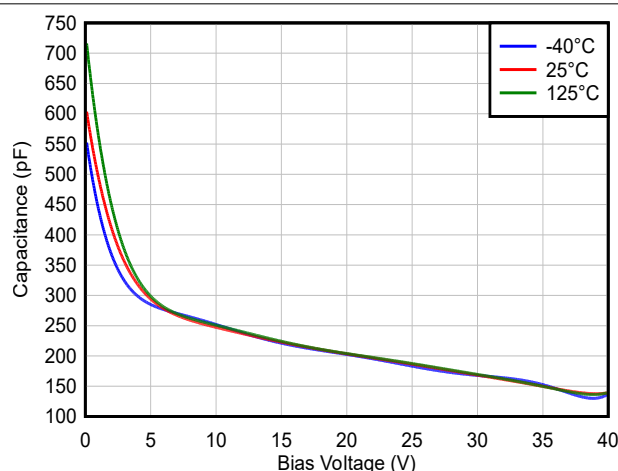
図 7-5. 温度範囲にわたる静電容量とバイアス電圧との関係
