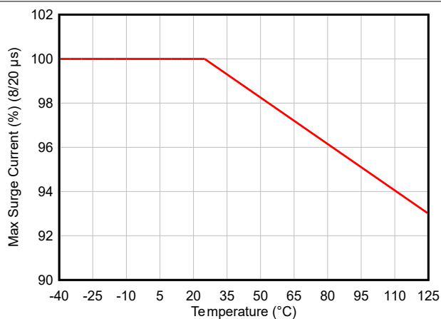
図 7-7. 最大サージ電流のディレーティング曲線
