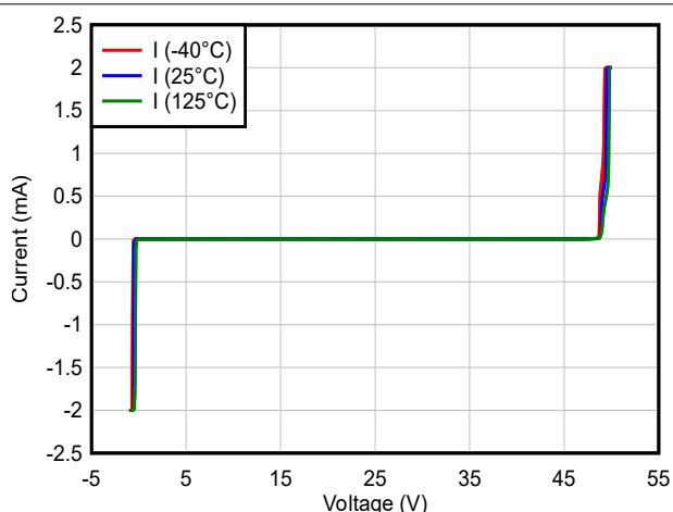
図 7-6. 温度範囲にわたる I/V 曲線
