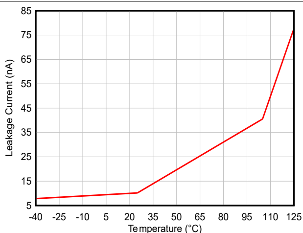
図 7-4. リーク電流と温度との関係
