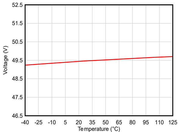
図 7-2. ブレークダウン電圧 (1mA) と温度との関係
