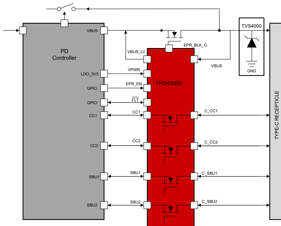
図 9-1. TVS4000 アプリケーション回路図
