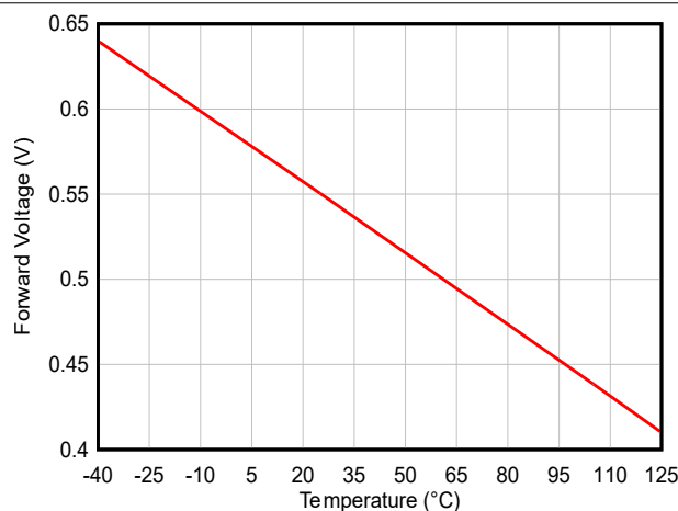
図 7-3. 順方向電圧と温度との関係
