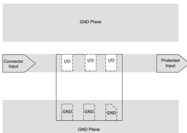
図 9-2. TVS4000DFN1616 のレイアウト
