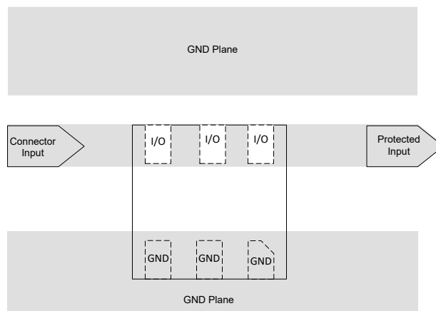
図 10-1. TVS5800DFN1616 のレイアウト
