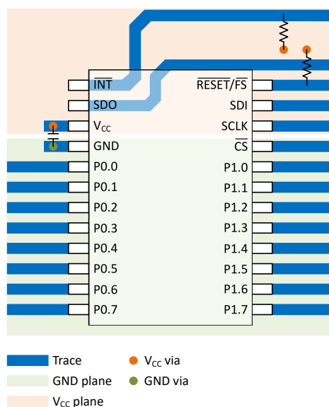
図 8-6. TXE8116-Q1 のレイアウト
