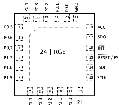
図 4-2. TXE8116-Q1 RGE (VQFN) パッケージ、24 ピン (上面図)
