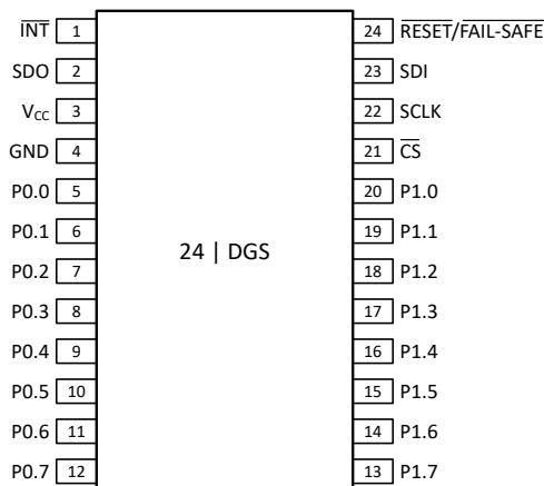
図 4-1. TXE8116-Q1 DGS (VSSOP) パッケージ、24 ピン (上面図)
