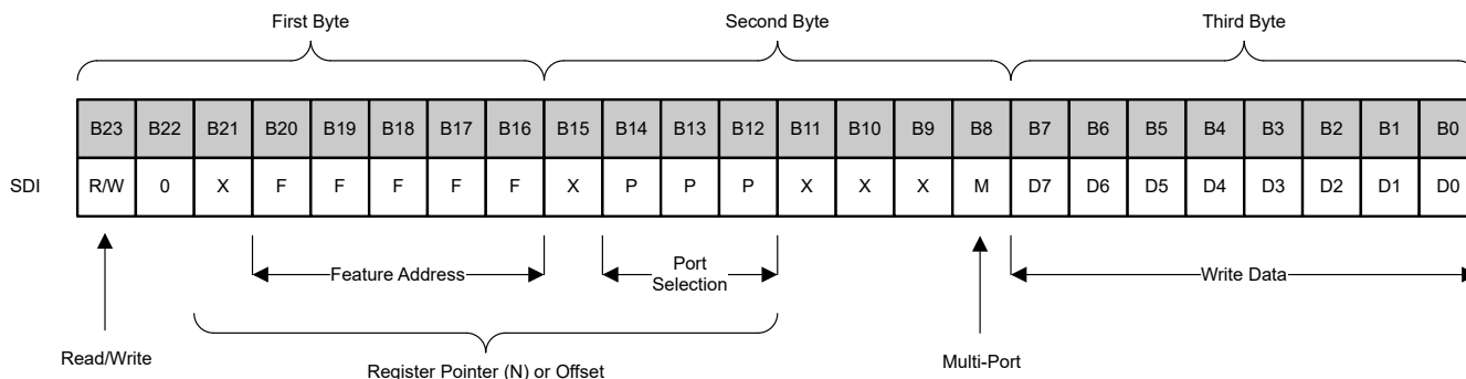
図 7-5. TXE8116-Q1 SPI SDI データ フレーム フォーマット
