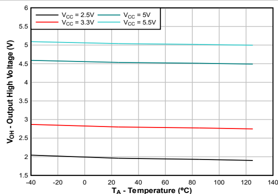
図 5-16. V_{OH} と温度の関係 - |I_{OH}| = 8\text{mA}
