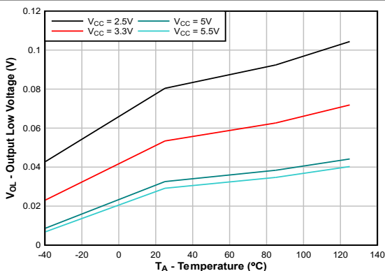
図 5-13. V_{OL} と温度の関係 - |I_{OL}| = 8\text{mA}
