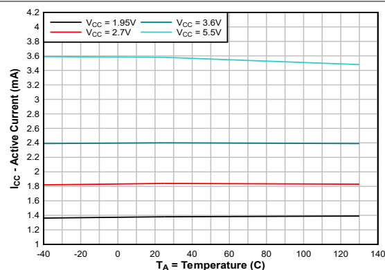
図 5-2. アクティブ電流と温度との関係 ( f_{\text{SCLK}} = 10\text{MHz} )
