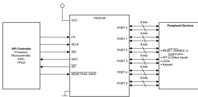
概略回路図
