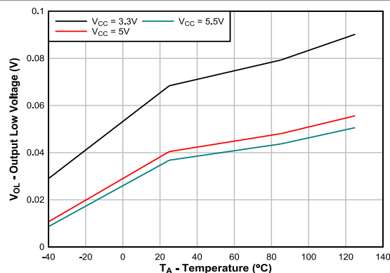
図 5-14. V_{OL} と温度の関係 - |I_{OL}| = 10\text{mA}
