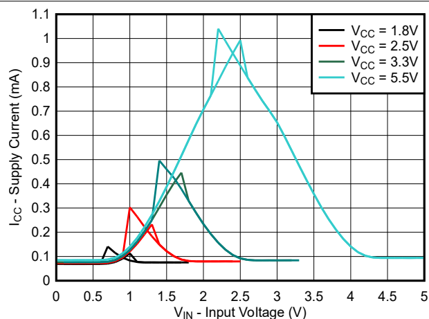
図 5-3. 電源電流 ( I_{CC} ) と入力電圧 ( V_{IN} ) との関係 [TXG0x010]
