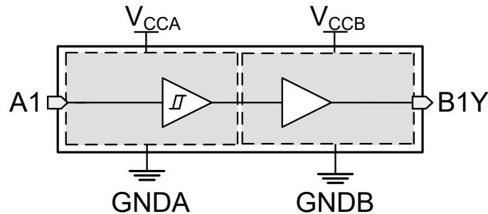
図 7-1. TXG1010 機能ブロック図
