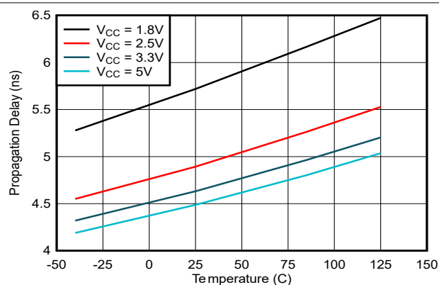
図 5-5. 伝搬遅延、 T_{PHL} 、と温度との関係
