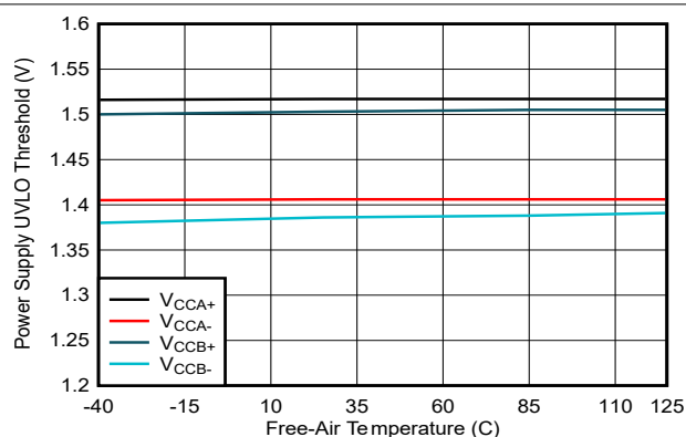
図 5-6. 電源低電圧スレッシュホールドと周囲温度との関係
