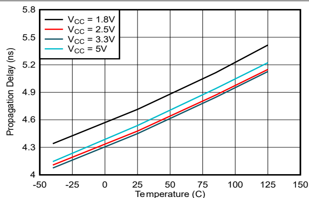
図 5-4. 伝搬遅延、 T_{PLH} 、と温度との関係
