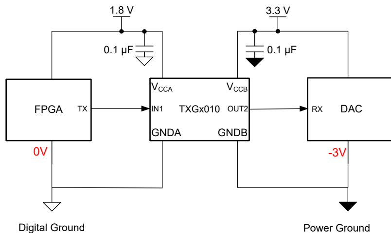
図 8-1. 試験および測定機器分野の TXG1010
