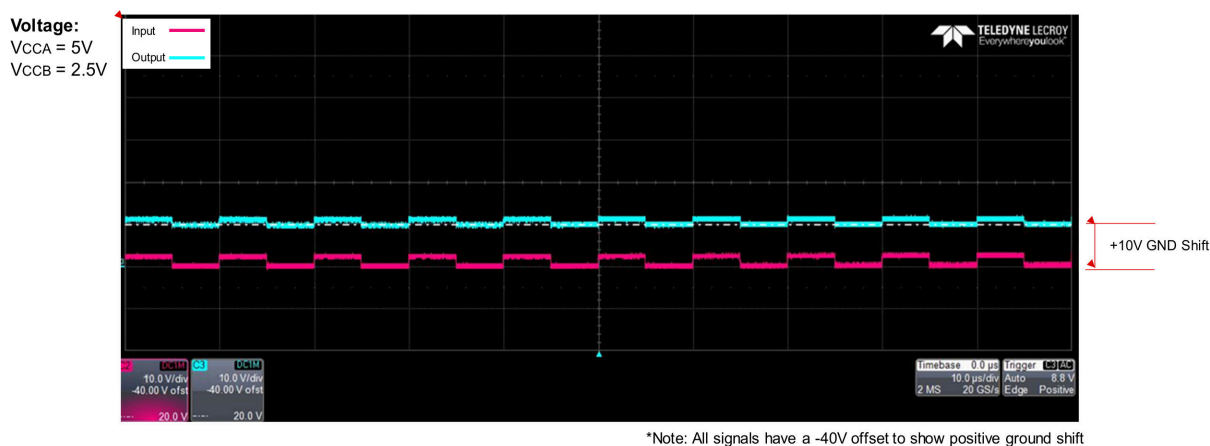
図 8-2. 5V から 2.5V への I/O 変換による -10V (上) および +10V (下) のグラウンドシフトを示す波形
