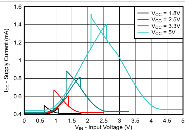
図 6-5. 電源電流 ( I_{CCA} ) と入力電圧 ( V_{IN} ) との関係 [TXG0x020]
