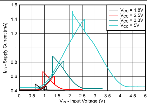
図 5-5. 電源電流 ( I_{CCA} ) と入力電圧 ( V_{IN} ) との関係 [TXGx020]
