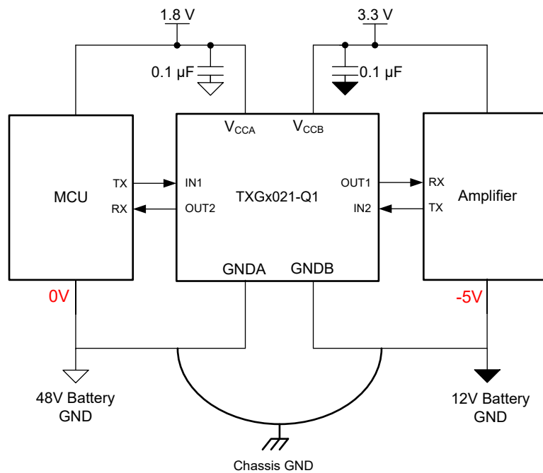
図 8-1. 車載用途での TXG4021-Q1
