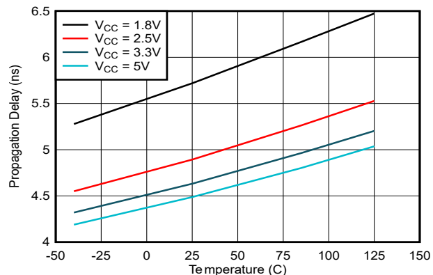
図 5-7. 伝搬遅延、T PHL 、と温度との関係
