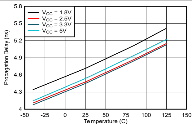
図 5-6. 伝搬遅延、 T_{PLH} 、と温度との関係
