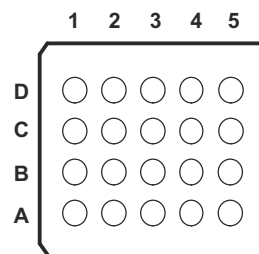
図 4-2. NME パッケージ、20 BGA (底面図)
