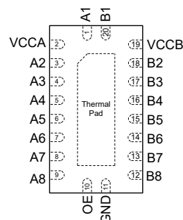
図 4-4. RKS パッケージ、20 ピン VQFN (上面図)
