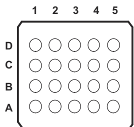
図 4-1. ZXY パッケージ、20 パンプ (底面図)
