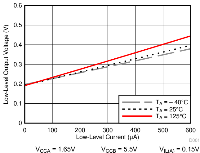
図 5-4. Low レベル出力電圧 ( V_{OL(Bx)} ) と Low レベル電流 ( I_{OL(Bx)} ) との関係
