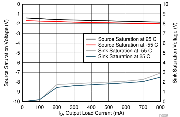
図 6-4. VCC = 15V、5ms の入力パルスでの OUTPUT 飽和電圧と負荷電流との関係
