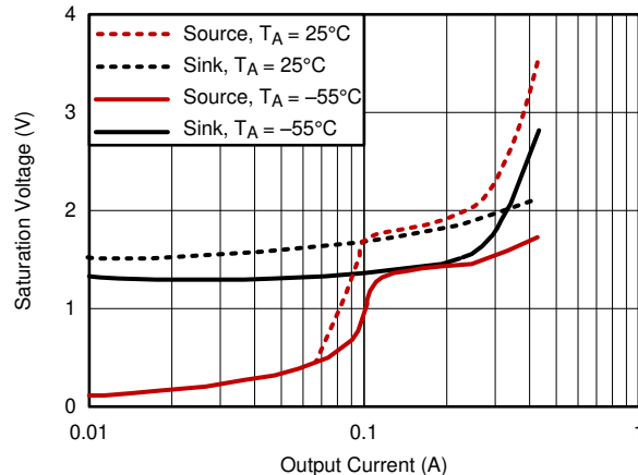
図 6-8. 出力飽和
