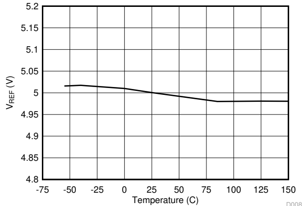
図 6-7. VREF 電圧と温度との関係
