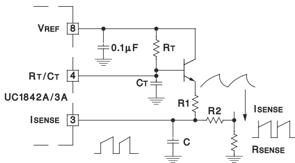
図 6-7. スロープ補償
