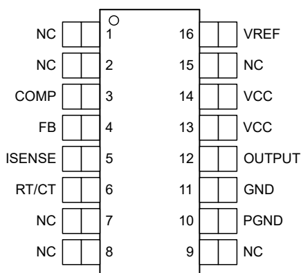
図 4-4. SOIC パッケージ、16 ピン DW (上面図)
