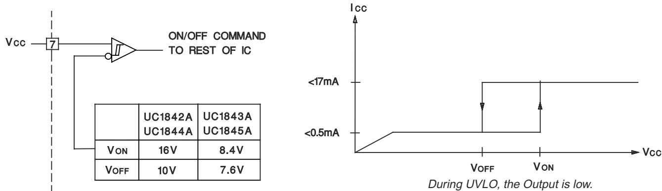
図 6-3. 低電圧誤動作防止
