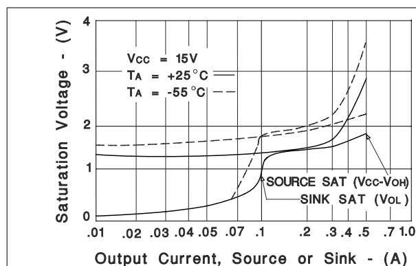
図 5-1. 出力飽和特性
