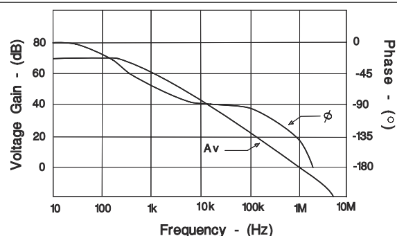
図 5-2. エラー アンプの開ループ周波数応答
