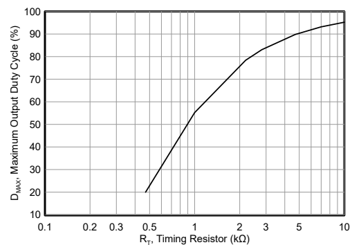
図 6-4. V_{CC} = 15V , C_T = 3.3nF , T_A = 25^\circ C での最大出力デューティ サイクルとタイミング抵抗との関係
