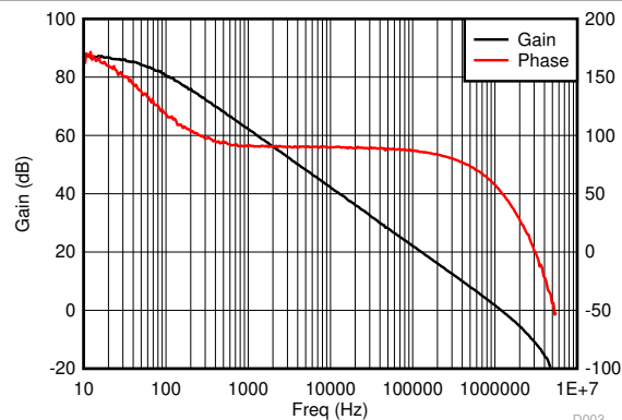
図 6-3. V_{CC} = 15V , R_L = 100k\Omega , T_A = 25^\circ C でのエラー アンプの開ループゲインおよび位相と周波数との関係
