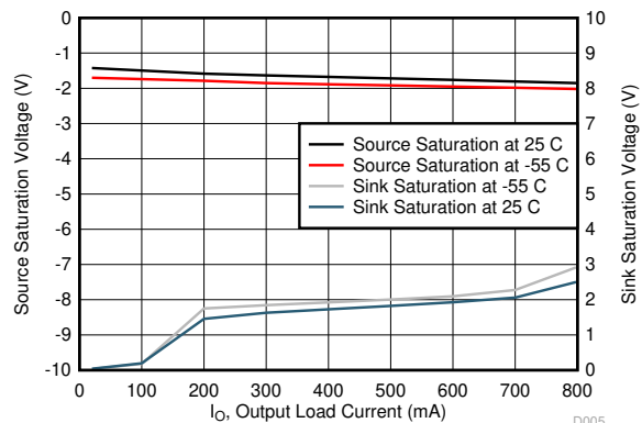
図 6-5. V_{CC} = 15V , 5ms 入力パルスでの出力飽和電圧と負荷電流との関係
