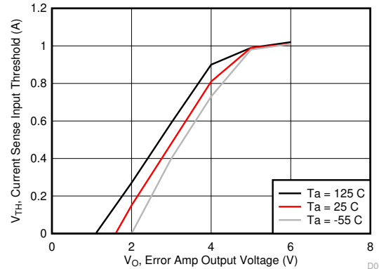
図 6-2. V_{CC} = 15V での電流センス入力レッシュリッドとエラー アンプ出力電圧との関係
