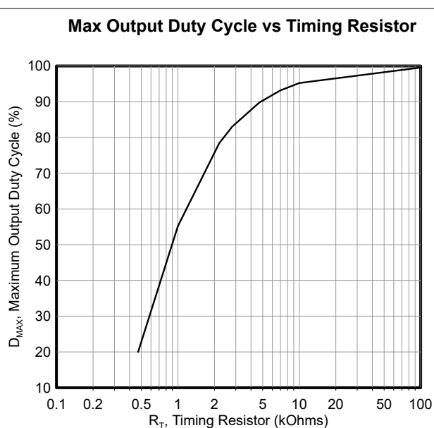
図 5-2. 最大デューティ サイクルとタイミング抵抗との関係
