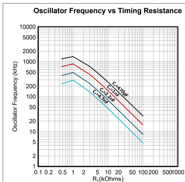
図 5-1. 発振器の周波数とタイミング抵抗との関係
