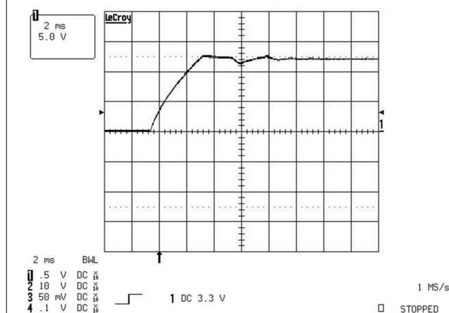
図 7-4. V_{OUT} スタートアップ全負荷
