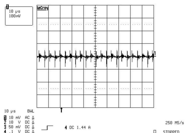
図 7-5. V_{OUT} リップル電圧
