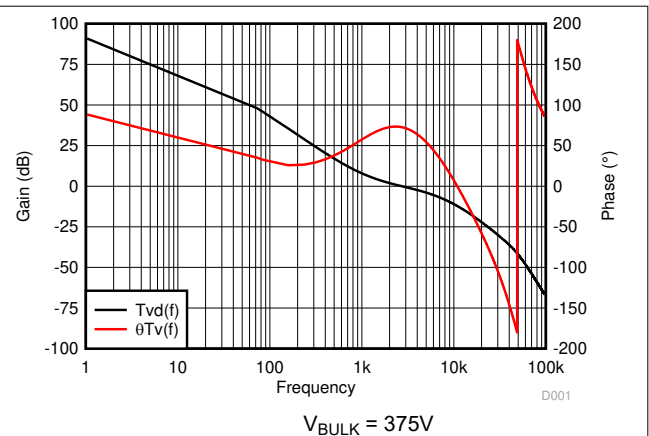
図 7-3. 電圧ループ・ゲイン
