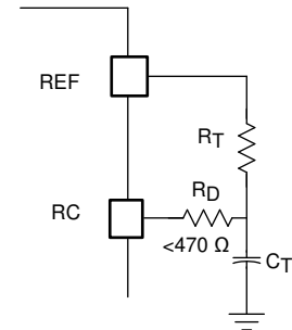
図 7-11. 制御された最大デューティ サイクルを生成する回路
