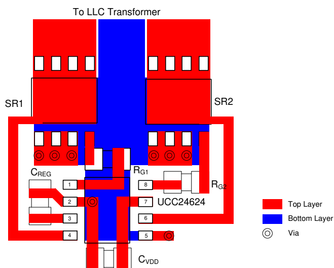
11-1. UCC24624 Layout Example
