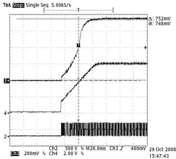
図 8-12. 標準的なソフト スタート波形
