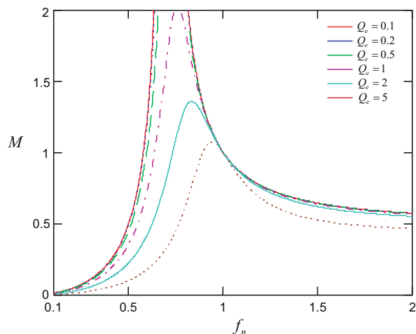
図 8-3. M と f_n との関係
