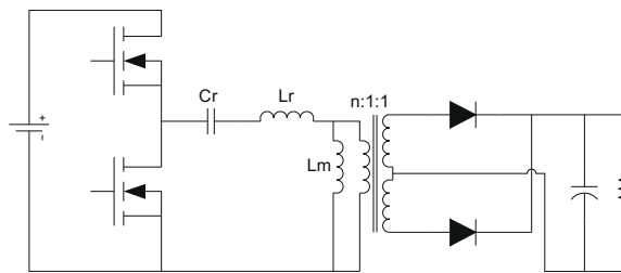
図 8-1. LLC 共振コンバータ
