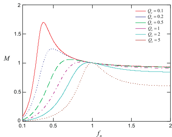
図 8-5. M と f_n との関係
