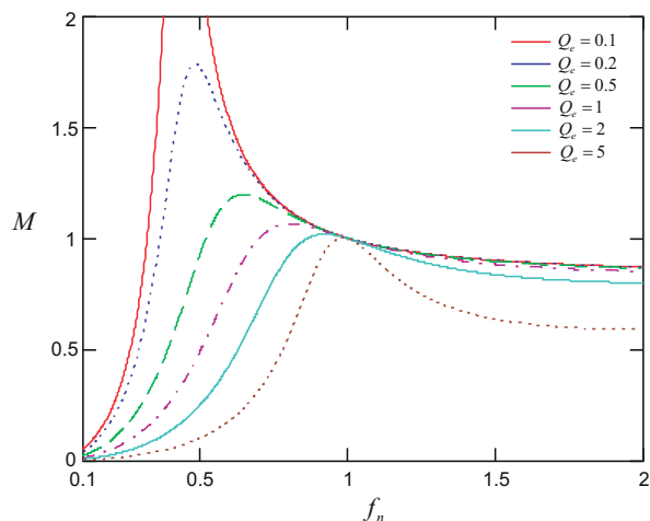
図 8-4. M と f_n との関係
