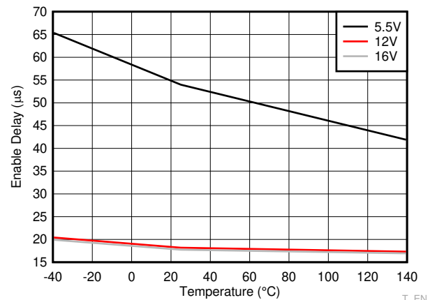
6-12. Enable Delay
