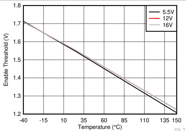
FIG 6-10. Enable Threshold
