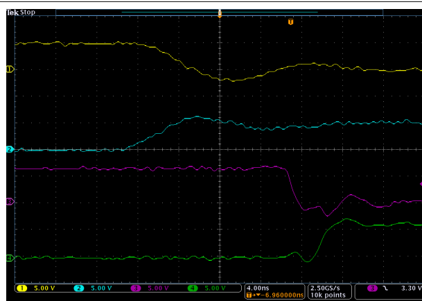
8-6. LO Fall Time
