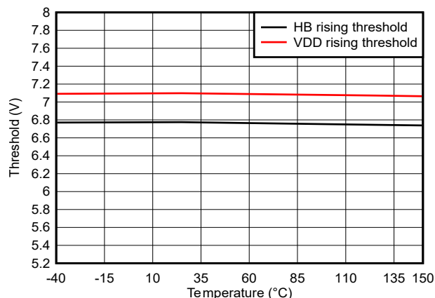
図 5-10. 低電圧誤動作防止スレッシュホールドと温度との関係
