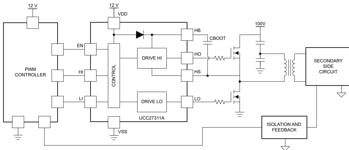
図 7-1. UCC27311A の代表的なアプリケーション図 1
