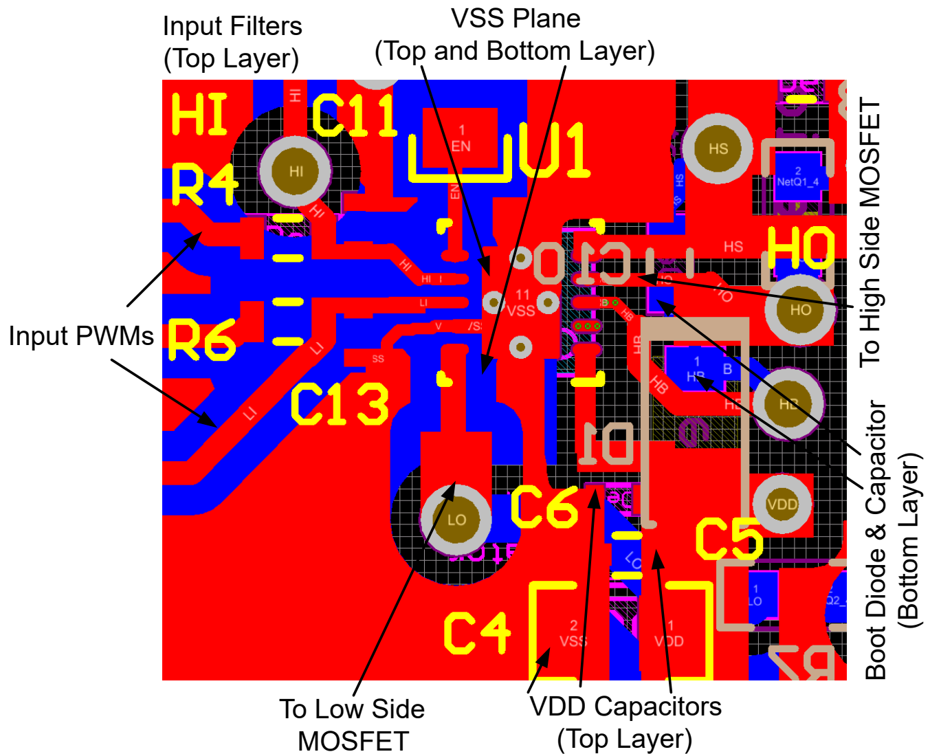
図 9-1. UCC27311A VSON パッケージの PCB レイアウト例
