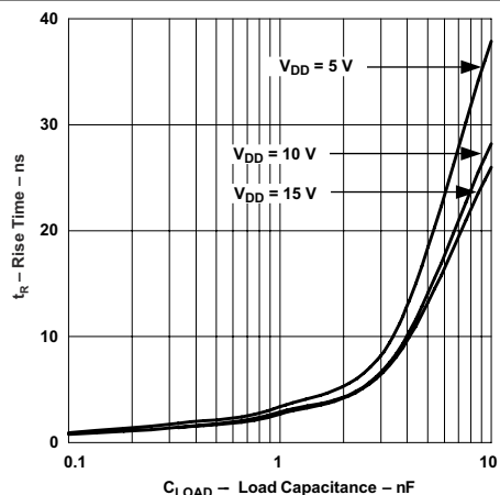
図 7-9. Rise Time vs Load Capacitance
