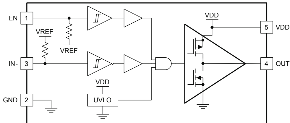
FIG 34. UCC27536
