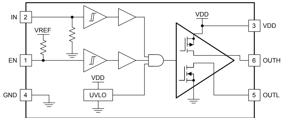
FIG 32. UCC27531
