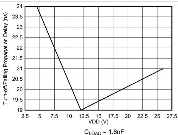
図 5-18. 入力から出力への立ち下がり (ターンオフ) 伝搬遅延と VDD との関係
