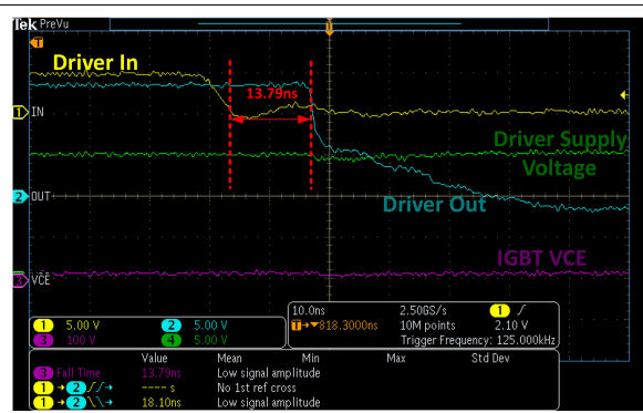
図 7-3. 昇圧コンバータの IGBT 駆動に使用されている UCC27624
