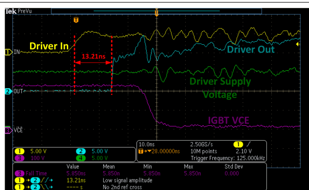
図 7-3. 昇圧コンバータの IGBT 駆動に使用されている UCC27624
