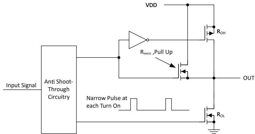
図 6-1. UCC27624 ゲート ドライバ出力構造
