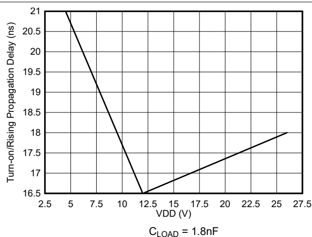
図 5-17. 入力から出力への立ち上がり (ターンオン) 伝搬遅延と VDD との関係
