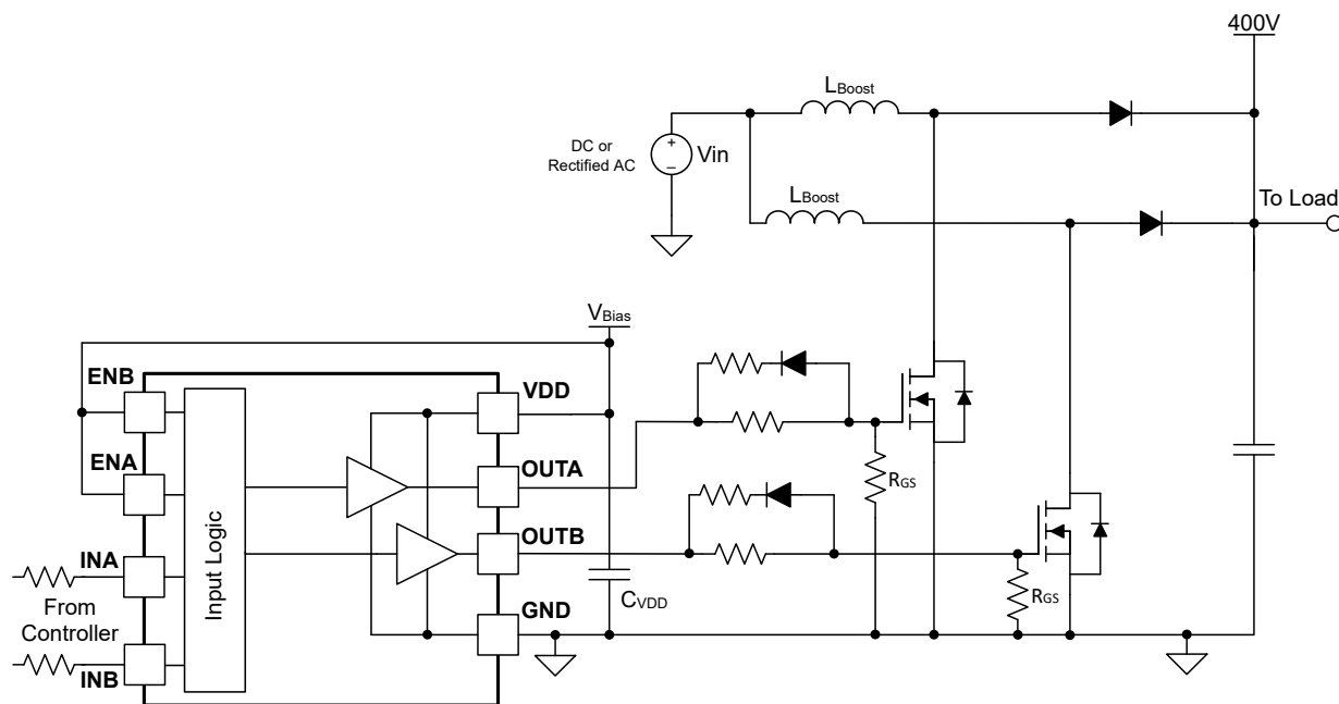
図 7-1. UCC27624 代表的なアプリケーションの図
