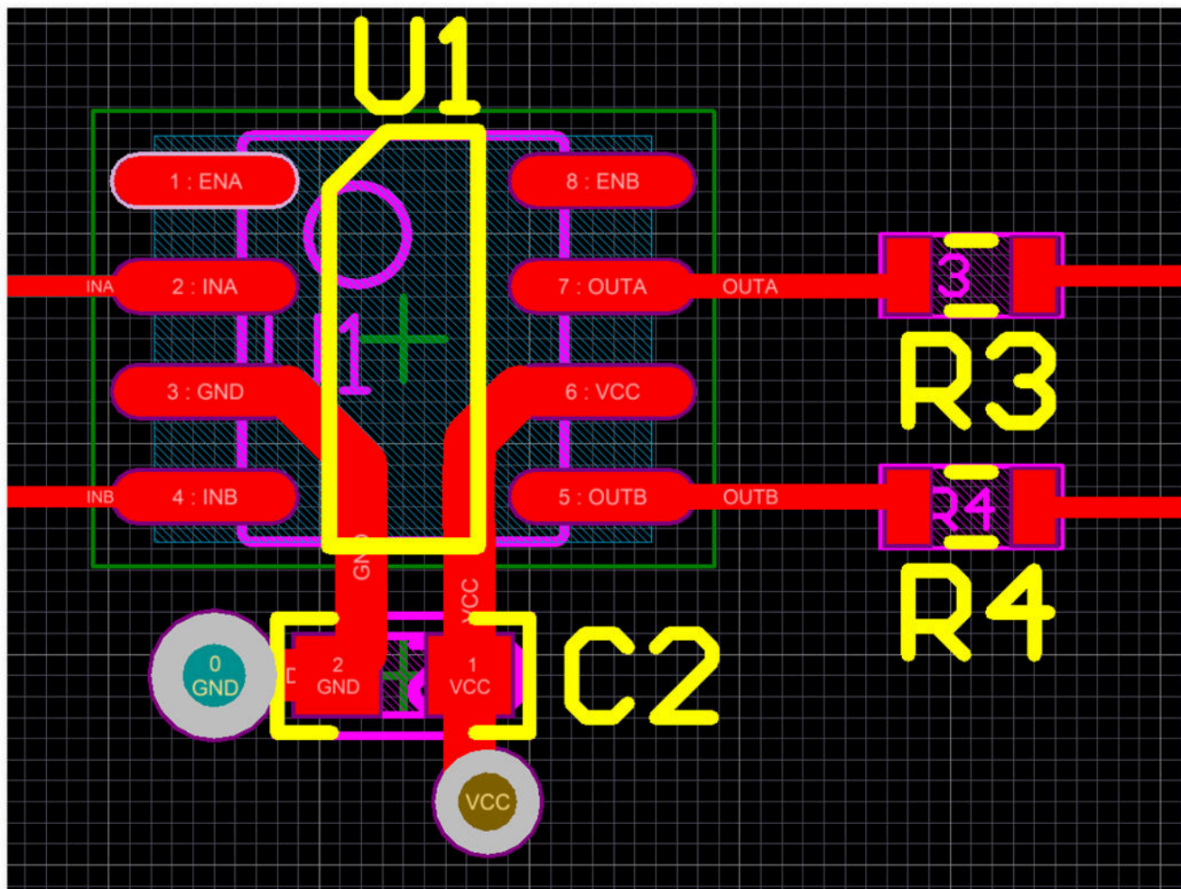
図 9-1. UCC27624 レイアウト例
