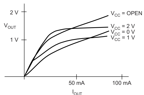
図 7-3. UVLO 中の OUT 電圧 vs OUT 電流
